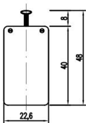
左视图 M1:1
